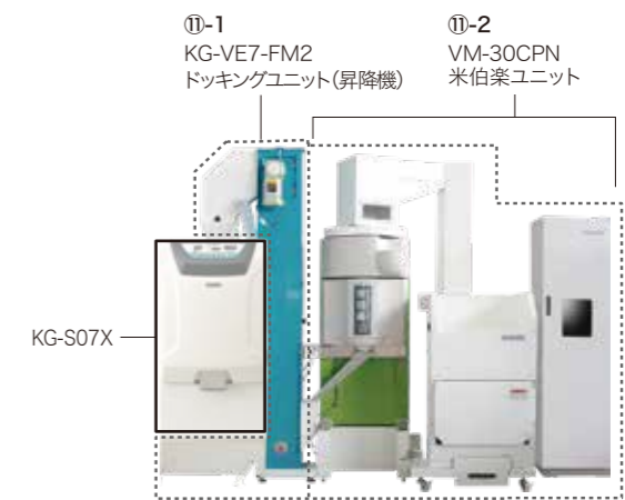
⑪ 3馬力精米ユニットVM-30CUPN
